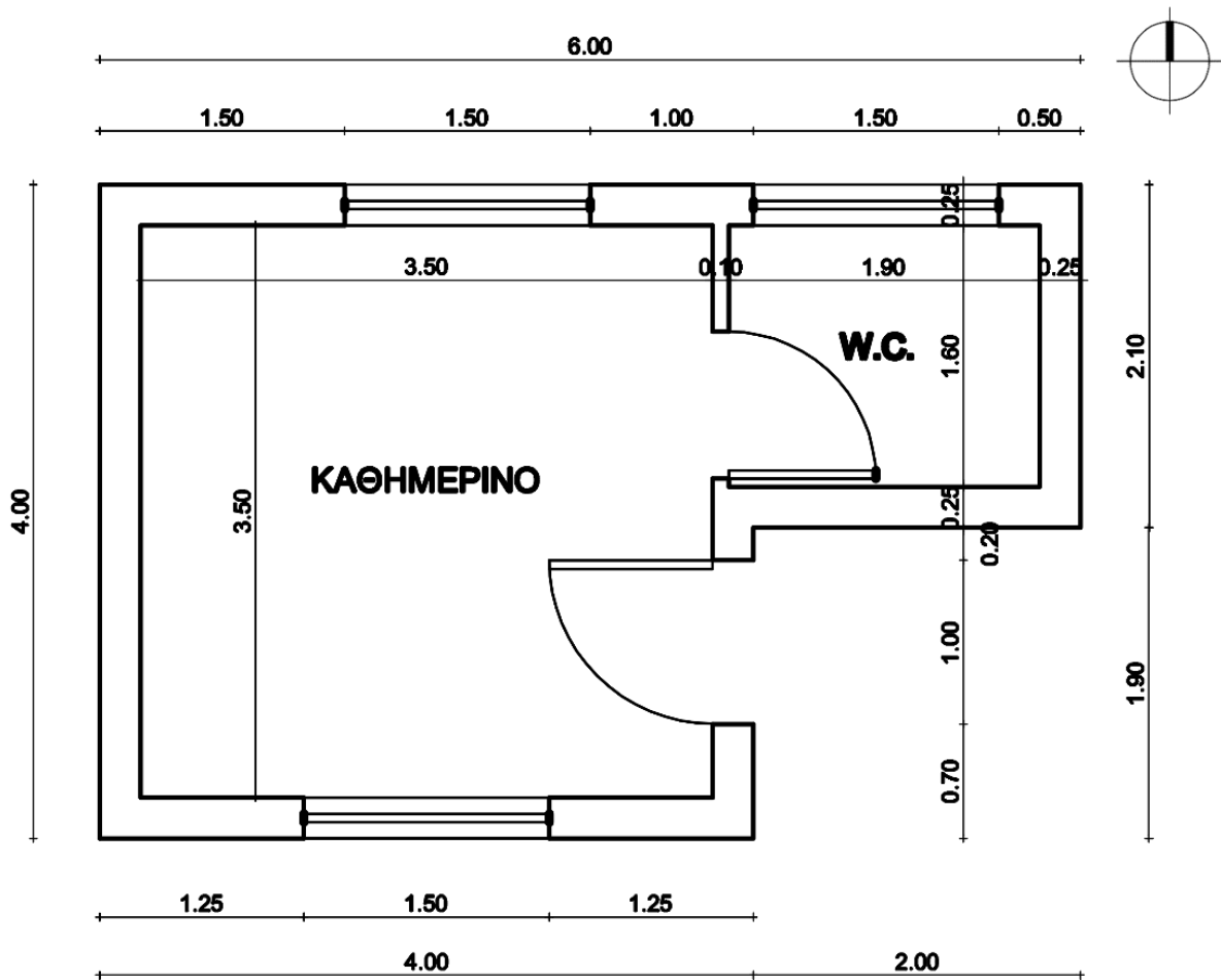
ΚΑΤΟΨΗ
